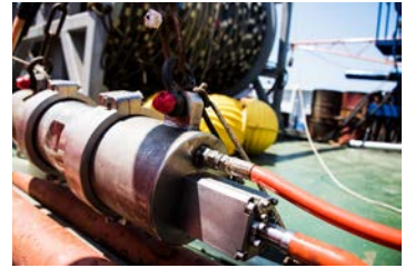
多頻道反射震測系統波源空氣槍
