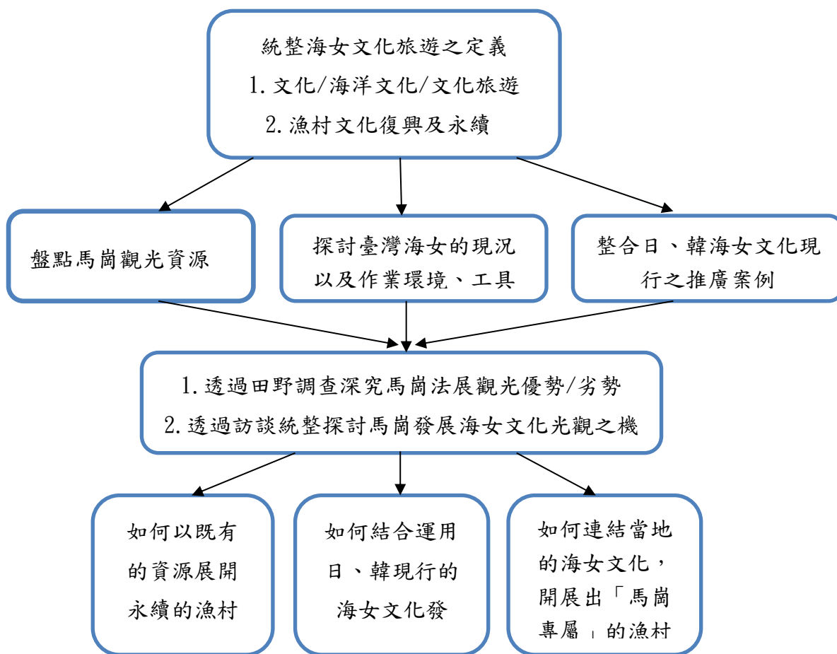
圖 2-2 研究架構圖
