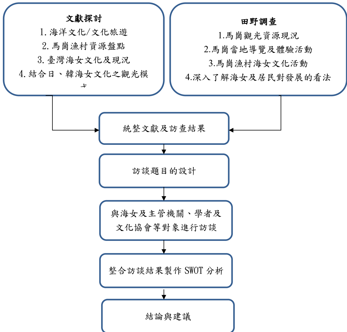
圖 2-3 研究流程圖
